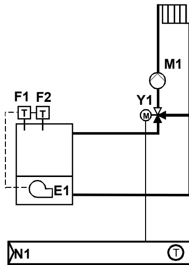
瞬間湯沸かし器 (温水暖房) 制御
