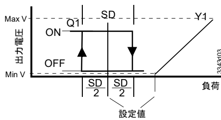
逆動作 (RA) + 正動作 (DA) ON/OFF + 比例 (アプリケーション 40-49)
