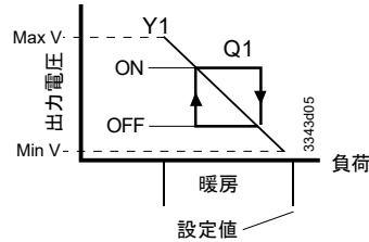
逆動作 (RA) x2 1 比例 + 1 ON/OFF (アプリケーション 20-29)
