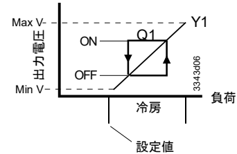
正動作 (DA) x2 1 比例 + 1 ON/OFF (アプリケーション 60-69)
