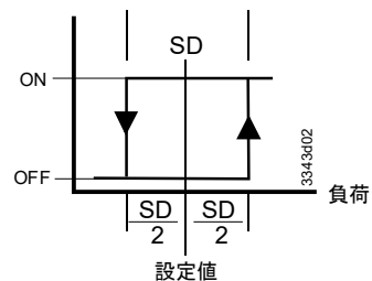
正動作 (DA) ON/OFF (アプリケーション 80-89)
