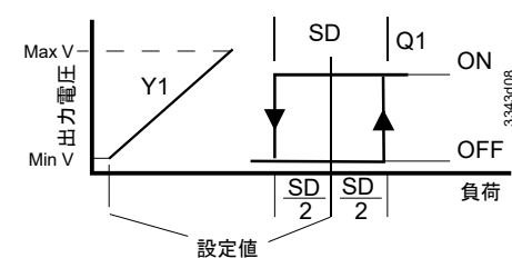
正動作 (DA) x2 1 比例 + 1 ON/OFF (アプリケーション 70-79)
