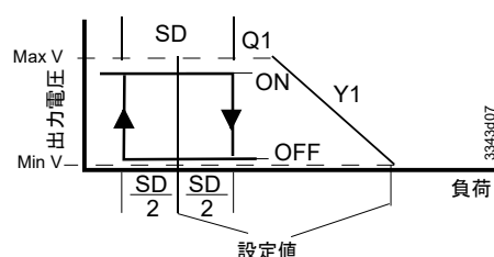
逆動作 (RA) x2 1 比例 + 1 ON/OFF (アプリケーション 30-39)
