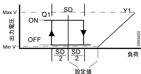
逆動作 (RA) + 正動作 (DA) ON/OFF + 比例 (アプリケーション 40-49)
