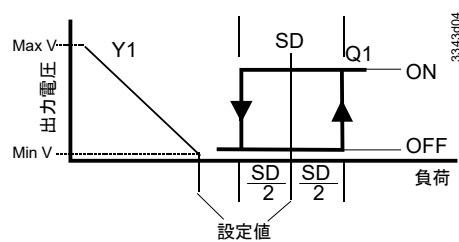
逆動作 (RA) + 正動作 (DA) 比例 + ON/OFF (アプリケーション 50-59)
