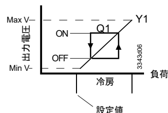
正動作 (DA) x2 1 比例 + 1 ON/OFF (アプリケーション 60-69)
