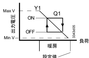
逆動作 (RA) x2 1 比例 + 1 ON/OFF (アプリケーション 20-29)
