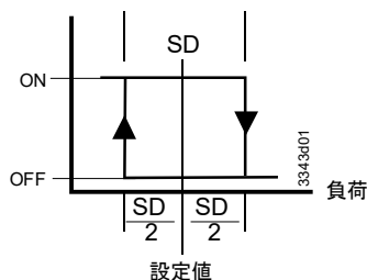
逆動作 (RA) ON/OFF (アプリケーション 10...19)
