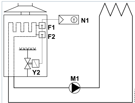
室内温度調節：ガス直焚き壁掛けボイラー制御
