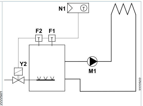
室内温度調節：ガス直焚き床置きボイラー制御
