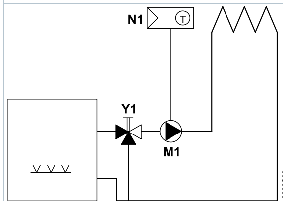
室内温度調節：温水循環ポンプ制御 (手動混合弁付き)
