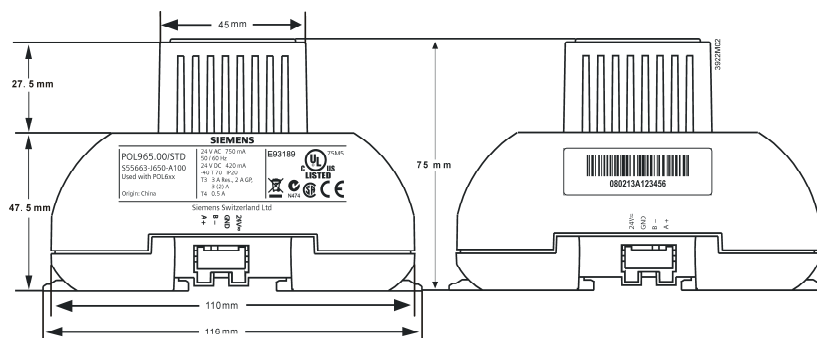
右側面
