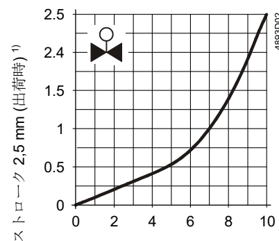
制御信号 Y [V]
