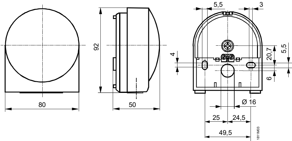
穴開け寸法
