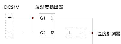
(温度計測のみ : G1-I1に電源が必要です)
