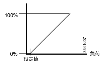
正動作 (DA) シーケンス (アプリケーション 70...79)
