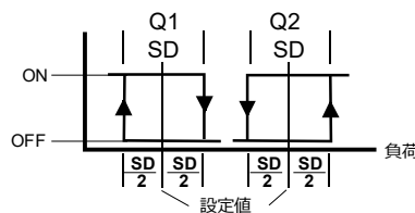
逆動作 (RA) + 正動作 (DA) (アプリケーション 40...49)
