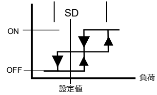
正動作 (DA)、ON/OFF x2 段 (連続ステップ) (アプリケーション 50...59)
