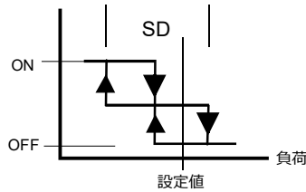
逆動作 (RA)、ON/OFF x2 段 (連続ステップ) (アプリケーション 10...19)
