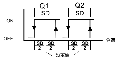
正動作 (DA)、ON/OFF x2 段 (独立ステップ) (アプリケーション 60...69)
