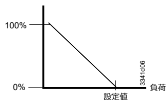
逆動作 (RA) シーケンス (アプリケーション 30...39)
