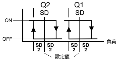
逆動作 (RA)、ON/OFF x2 段 (独立ステップ) (アプリケーション 20...29)
